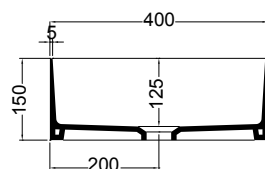
SEZIONE
